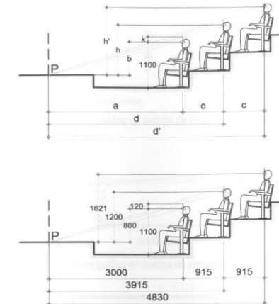
Sistema matemático para hallar las visuales verticales - Figura 01 Manual de estándares para la intervención de teatros
