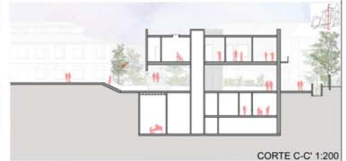
CORTE C-C' 1:200
