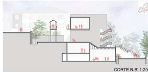
CORTE B-B' 1:200
